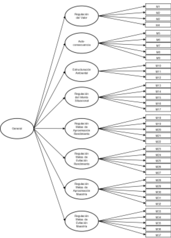
Figura 4 Modelo 4 ESEM
