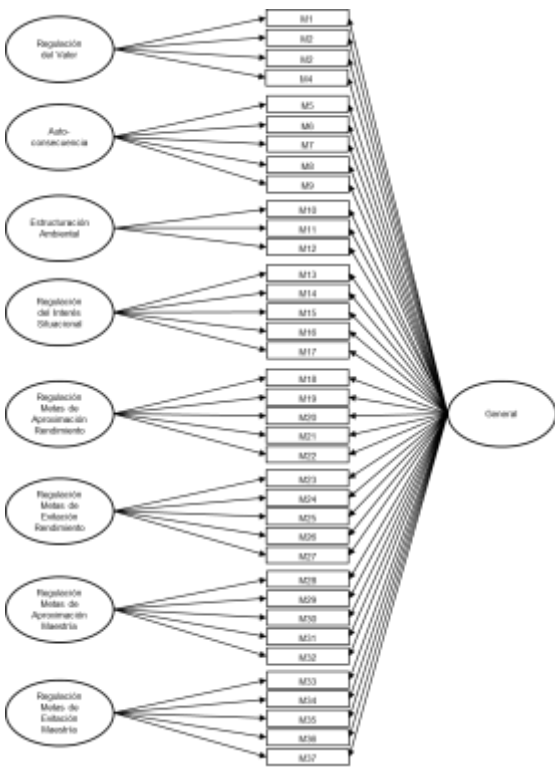
Figura 3 Modelo 3 bifactor
