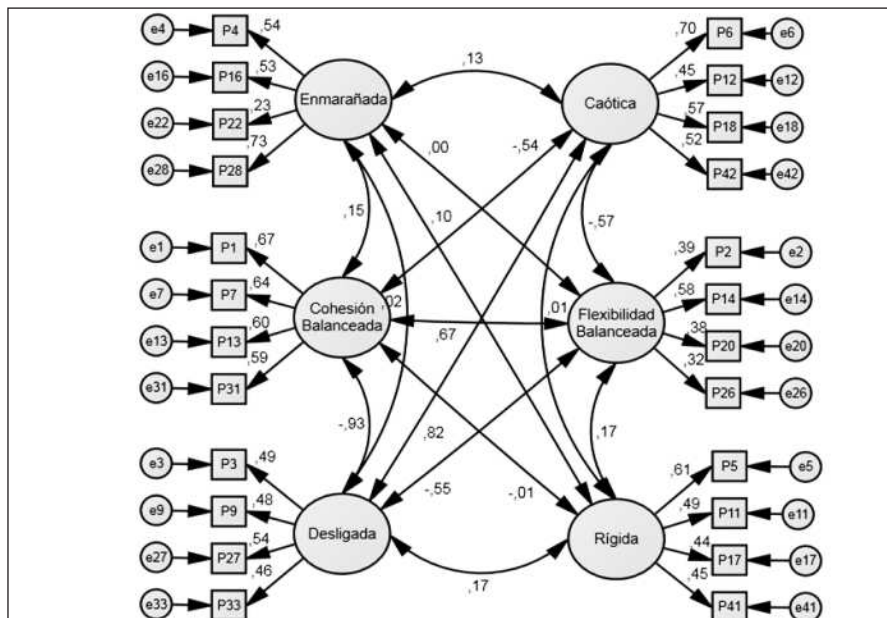
Figura 1. Resultados del análisis factorial confirmatorio para el FACES IV (usando el paquete estadístico AMOS)
